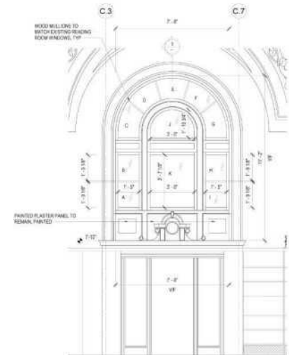
Plano de la ventana del arquitecto Biblioteca de la sucursal de la Misión
